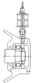
Fig. 12.5 Lubricación por Goteo de Aceite
