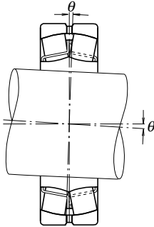
Fig. 3.4 Desalineación permisible de los rodamientos de rodillos esféricos
