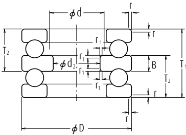
Fig. 7.4 Rodamientos de Bolas de Empuje de Doble Dirección
