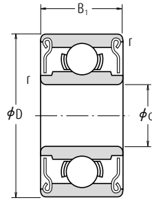
Tipo Blindado ZZ · ZS
