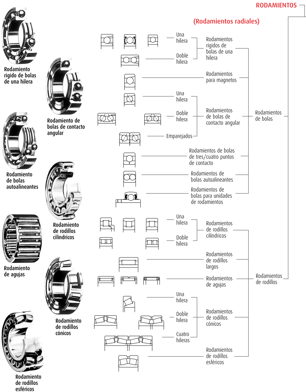
Fig. 1.2 Clasificación de Rodamientos
