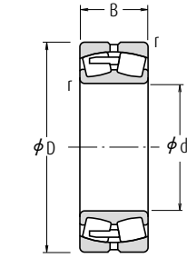
Diámetro Interior Cilíndrico
