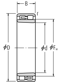
NNU Diámetro Interior Cónico
