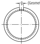
(Geometría del anillo elástico de posicionamiento encajado en la ranura)
