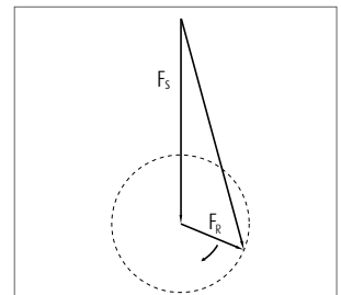
Fig. 5.10 Carga giratoria y carga estacionaria
